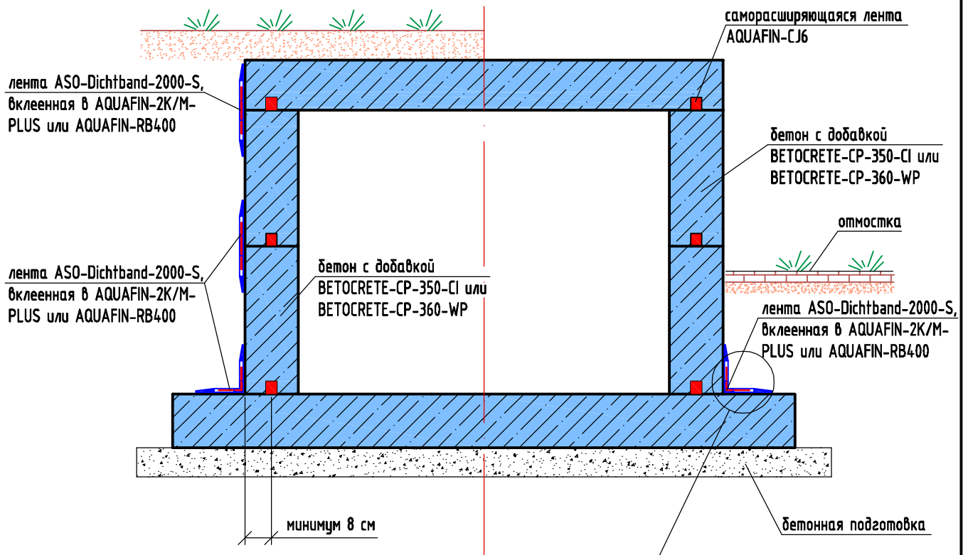
Альтернативный вариант устройства стыка
