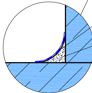
Альтернативный вариант устройства стыка
